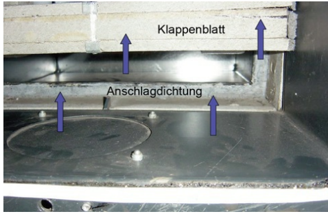
Serranda tagliafuoco, Carbotech
